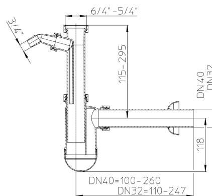
Чертёж HL132.1
