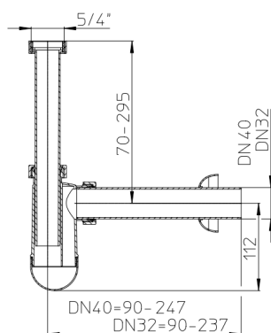
Чертёж HL132
