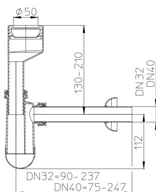
Чертёж HL130
